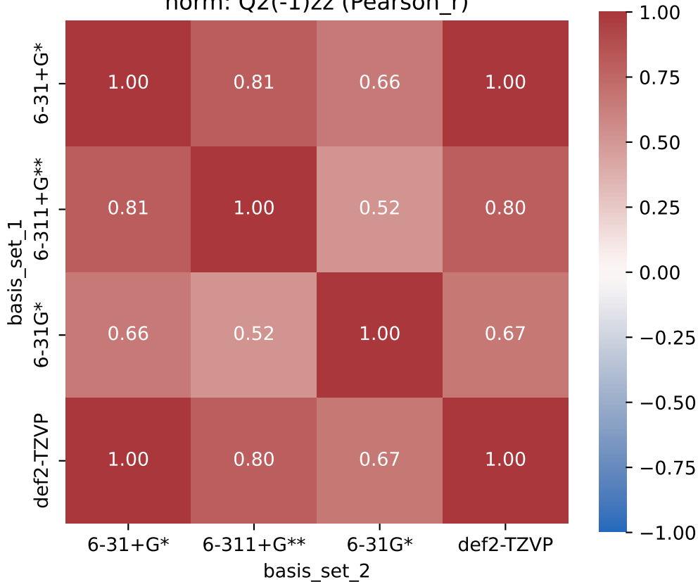
norm: Q2(-1)zz (Pearson_r)
